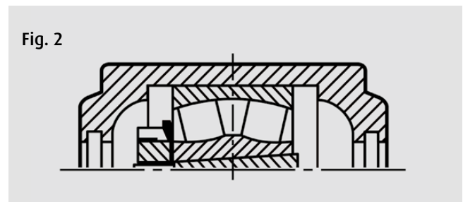
Fig.2 : Le palier libre doit permettre le déplacement axial du roulement dû à la dilatation axiale de l'arbre. Ce palier ne doit pas être équipé de bagues d'arrêt.
