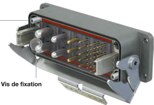
Broches de codage
