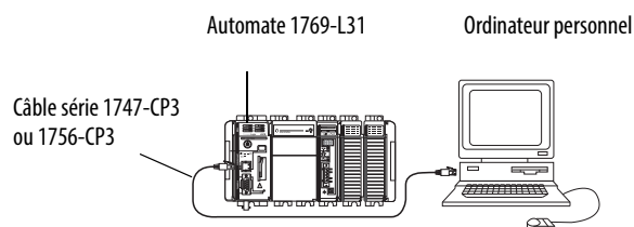
Figure 3 – Connexion série à l'automate
