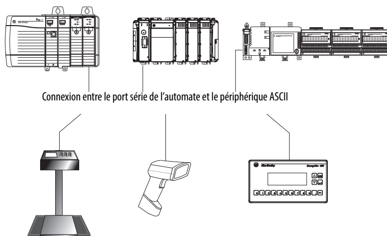
Figure 8 – Communication série avec des dispositifs ASCII
