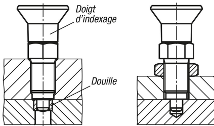
Fixation avec douille :
