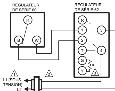
Fig. 6 — Raccordement d'un servomoteur de série 61
