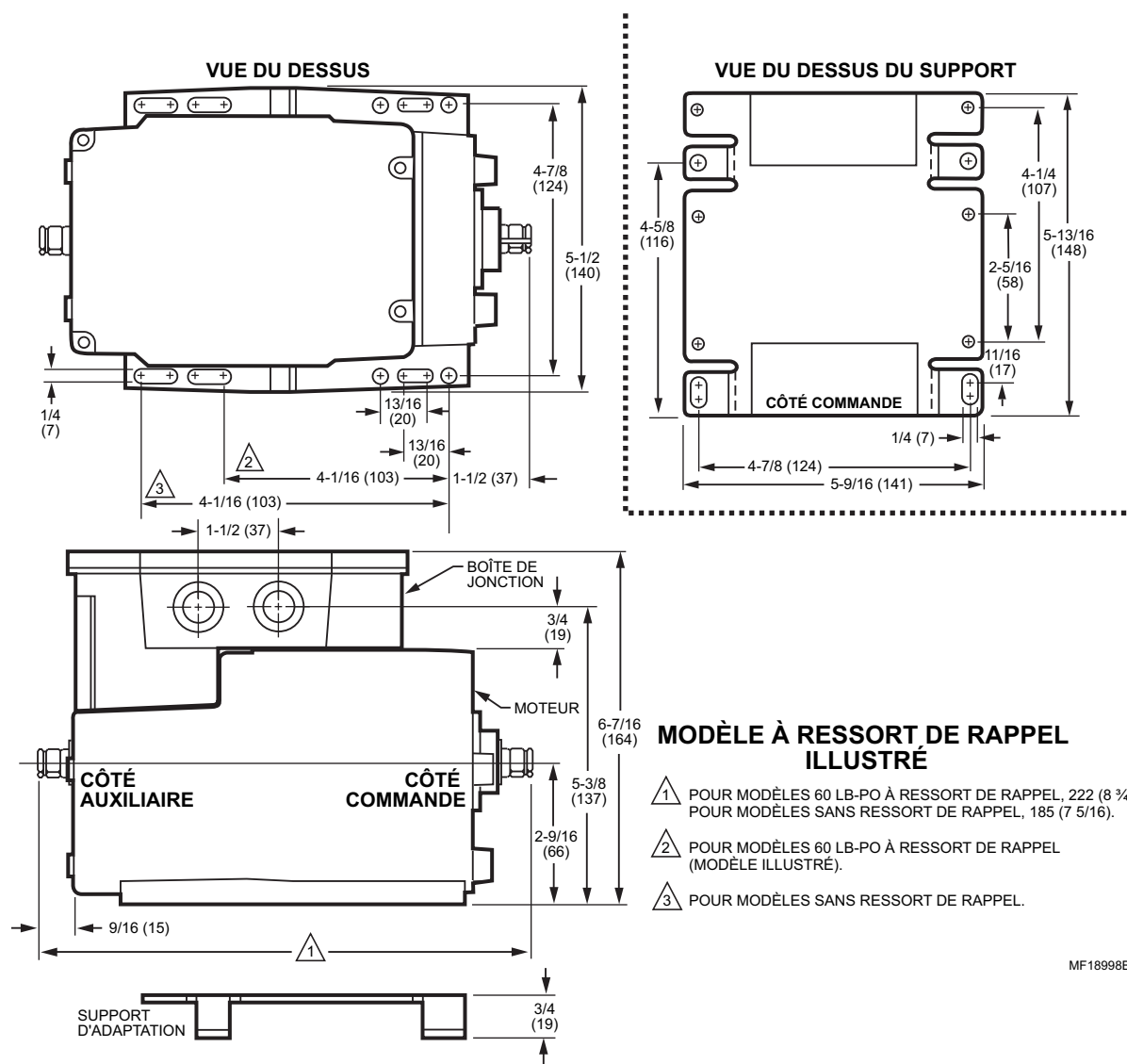
Fig. 1— Encombrement des servomoteurs Modutrol IV de séries 61 et 62 en po (mm).
