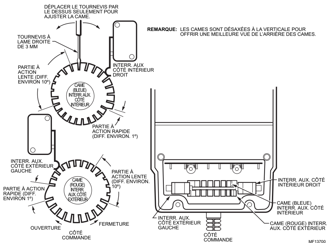
Fig. 14— Réglage de l'interrupteur auxiliaire.
