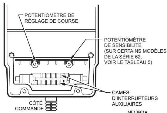
Fig. 12 — Configuration des réglages de la course
