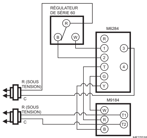
Fig. 10 — Raccordement de moteur asservi de série 90 ou de série 60
