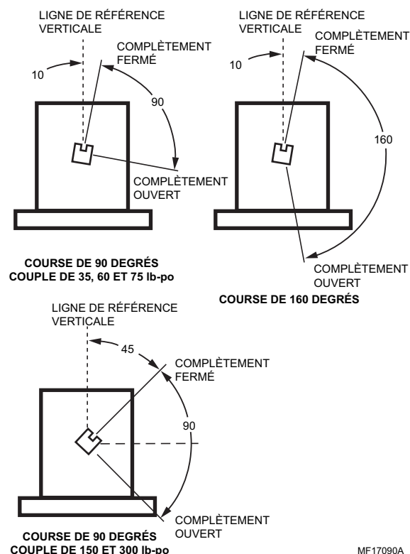
Fig. 2 — Positions de l'arbre du servomoteur aux limites de la course (vu du côté commande du servomoteur).
